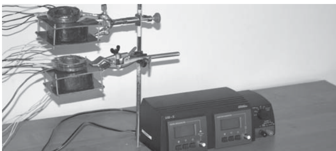
Лабораторный макет установки по электромагнитной обработке рудного сырья для увеличения извлекаемости полезных ископаемых в микро- и субмикро объемах
